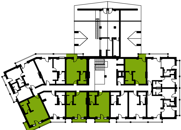
Potkrovlje Ukupno jedinica tipologije A1 u potkrovlju: 5
