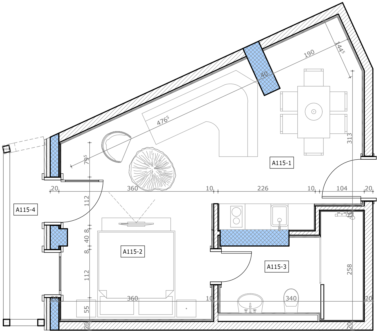
Prizemlje Ukupno jedinica tipologije A4 u prizemlju: 0
