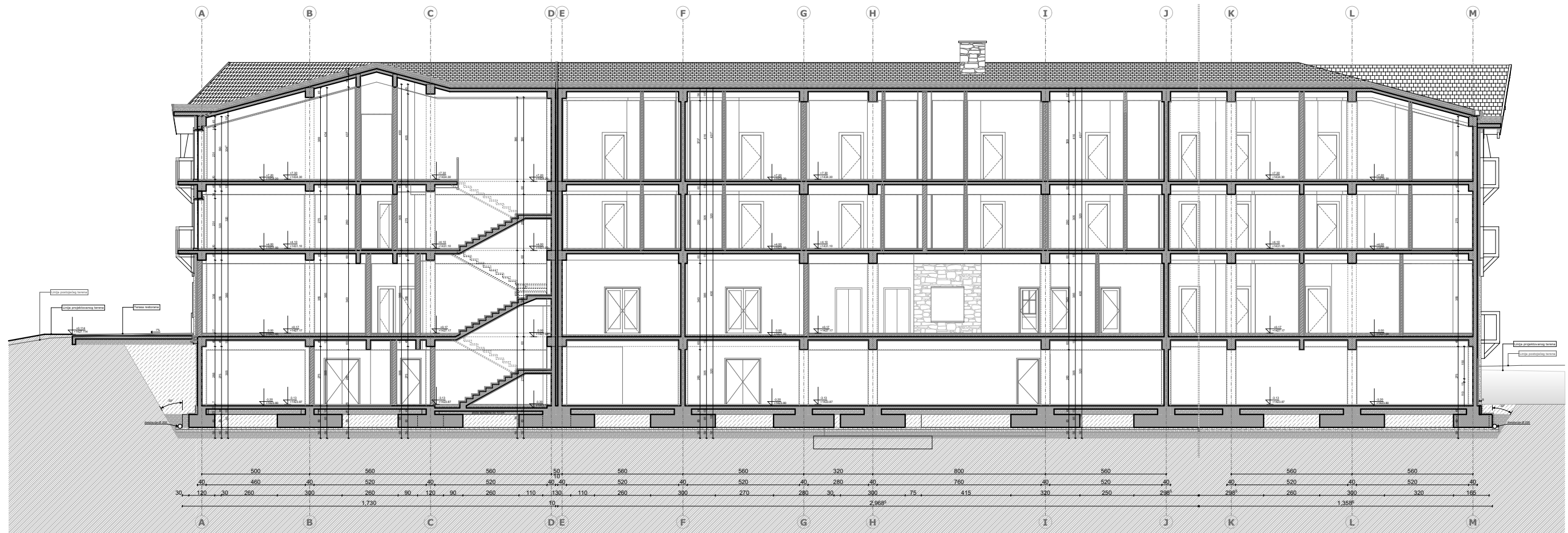
Presjek 2-2
