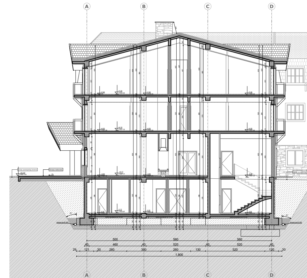
Presjek 3-3
